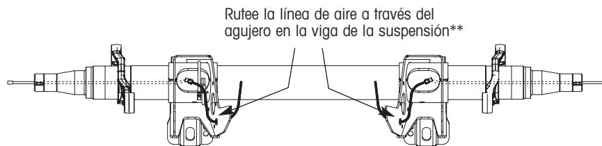
Figura 25. Detalles de instalación sugerida de la línea de control para Modelos Estándar de Perfil Bajo, Viga Corta, Buje Angosto (AANLS 20K)
