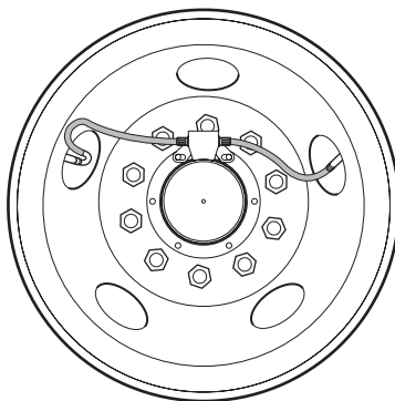
Configuración de llanta dual Orientación "B"
