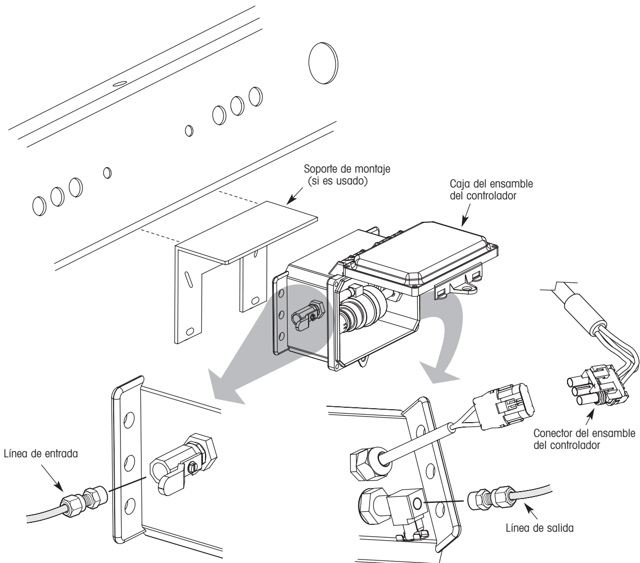
Figura 37. Reemplazo del ensamble del controlador
