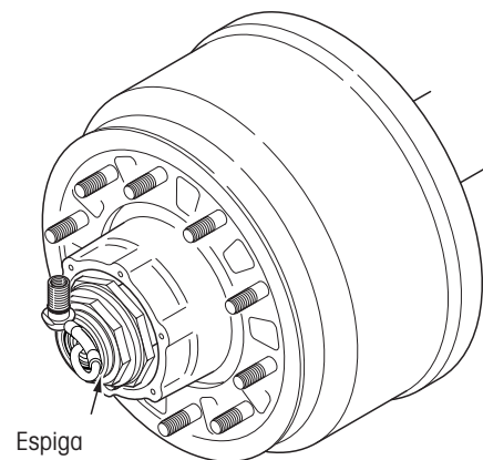
Figura 17. Ensamble de la junta rotativa instalado
