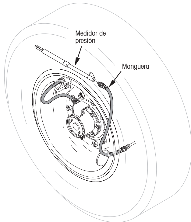
Figura 1. Revisión manual de presión en llantas
