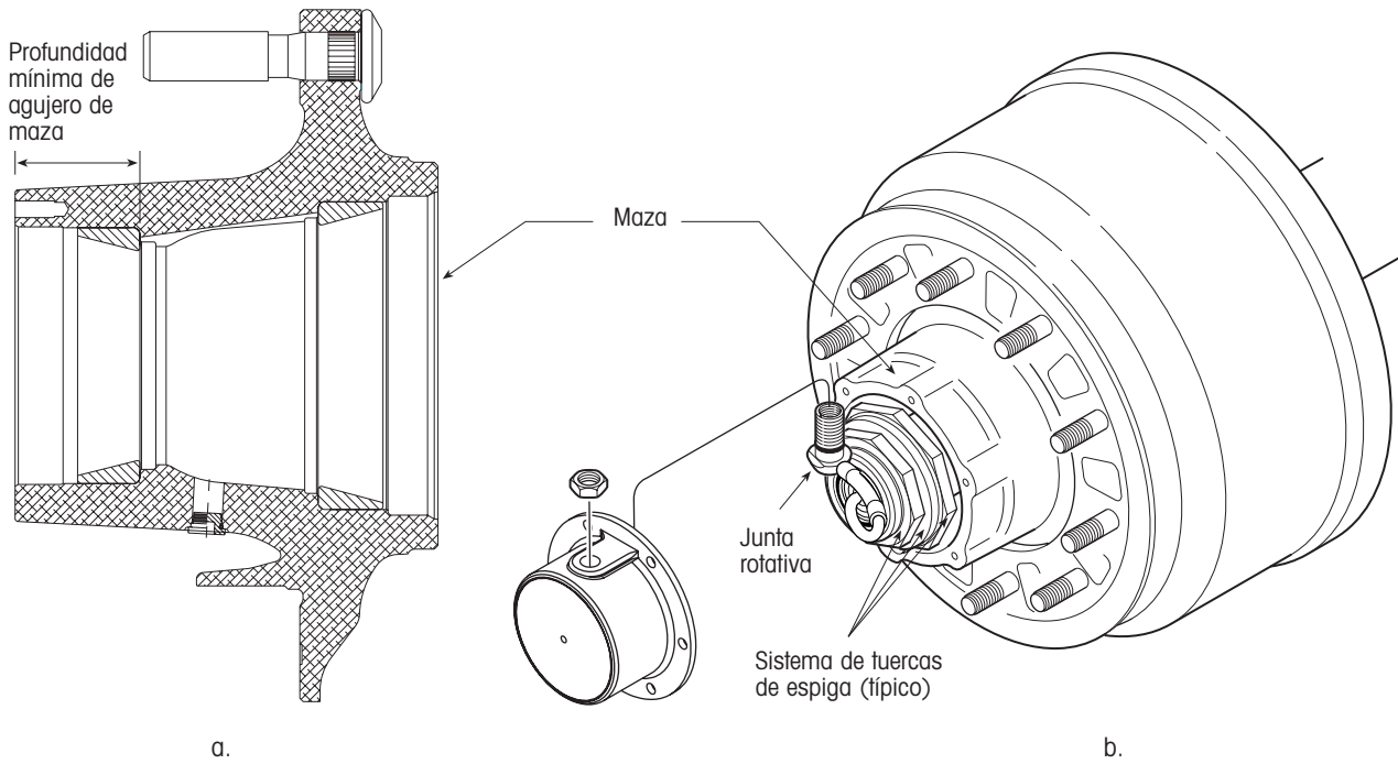
Figura 11. Requerimientos de maza para TIREMAAX® CP
