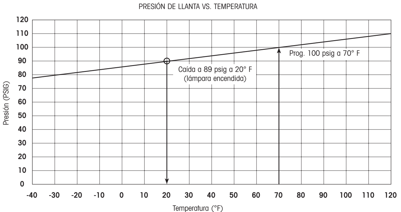
Figura 41. Desempeño típico del sistema de inflado de llantas a 100 psig
