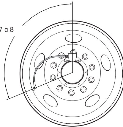
Configuración de llanta sencilla ancha
