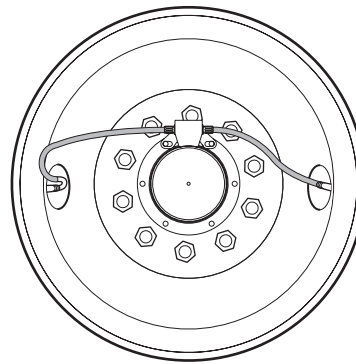
Configuración de llanta dual Orientación "C"
