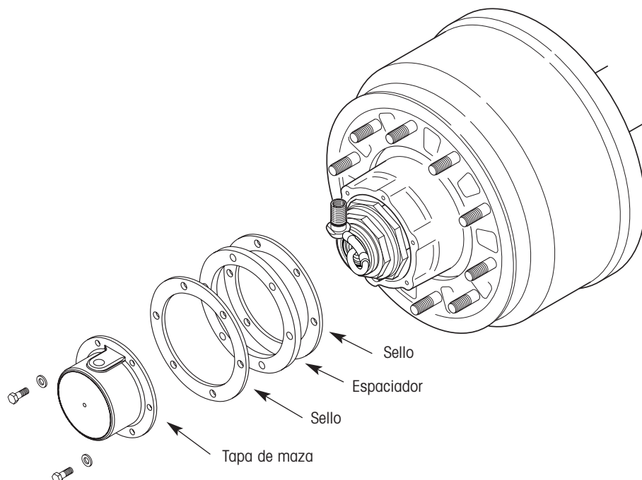
Figura 13. Instalación del kit de espaciador de tapa de maza
