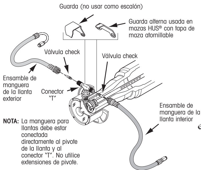
Configuración de llantas duales
