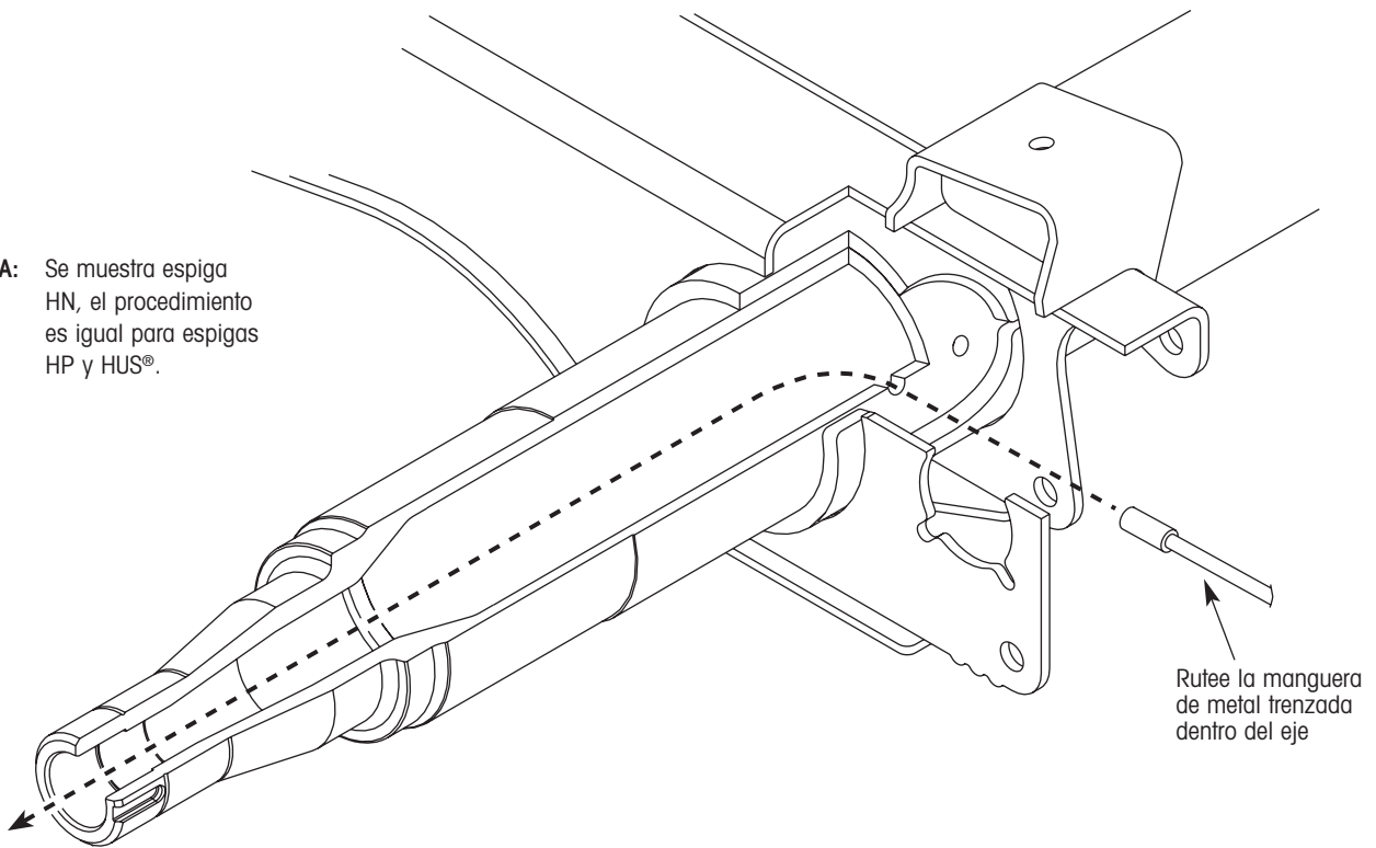
Figura 8. Ruteo de la manguera en el eje
