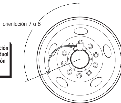
Configuración de llanta sencilla ancha
