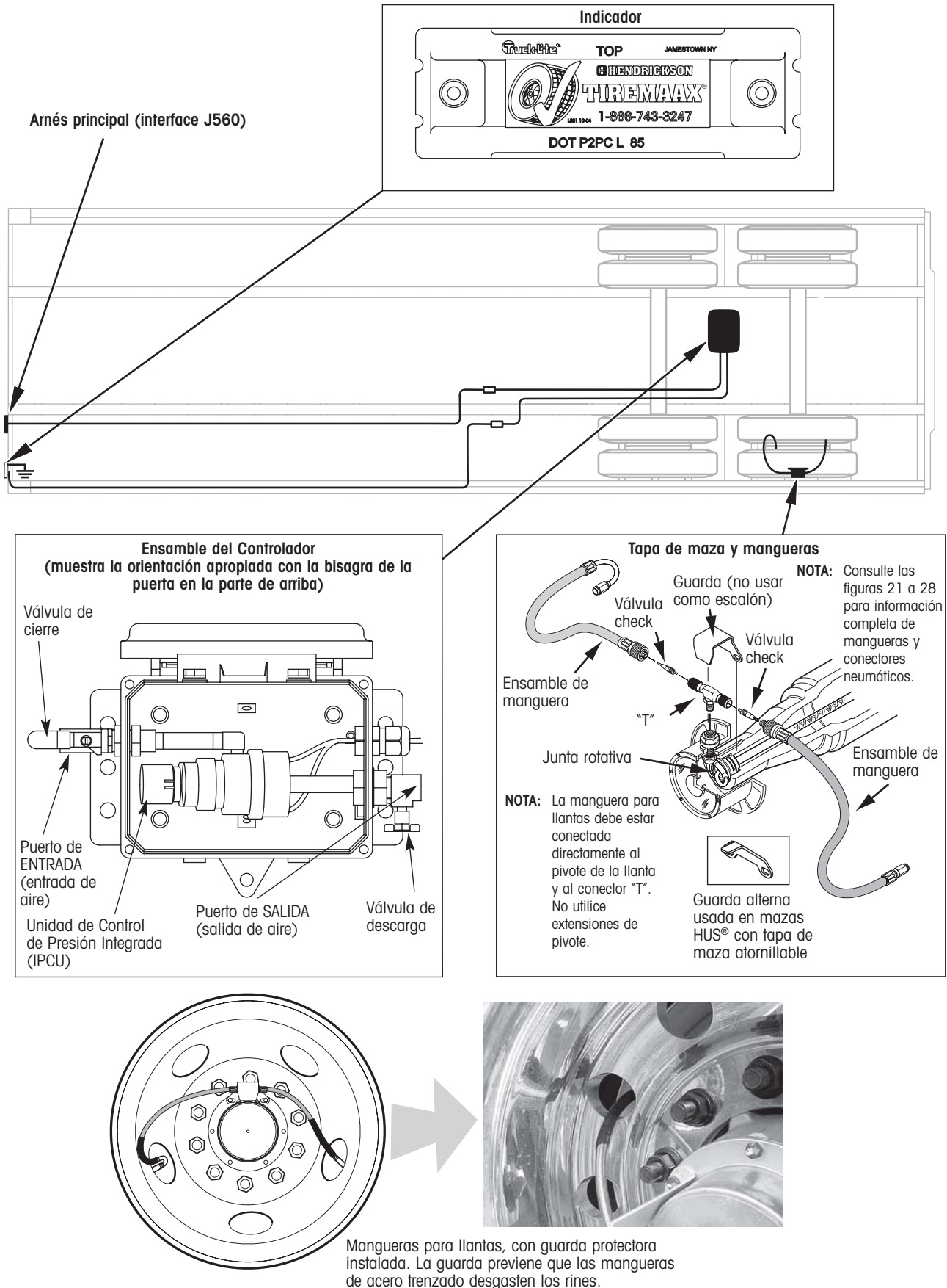
Figura 3. Componentes de TIREMAX® CP
