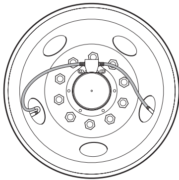
Configuración de llanta dual Orientación "A"
