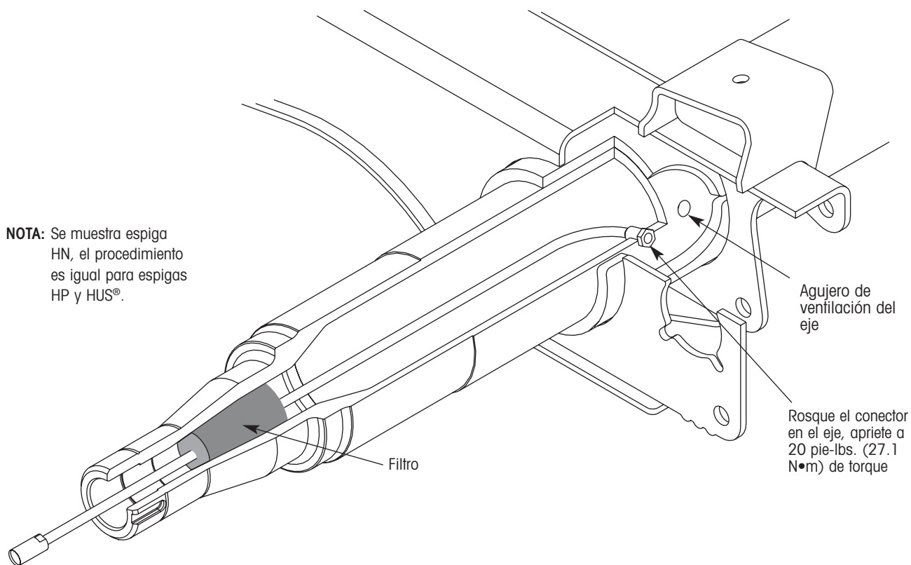
Figura 9. Manguera para eje instalada
