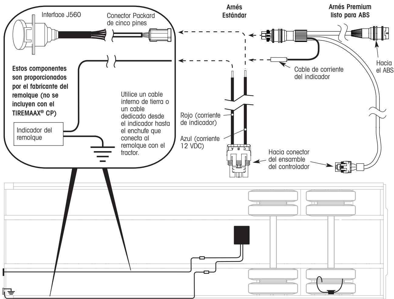
Figura 20. Instalación del arnés
