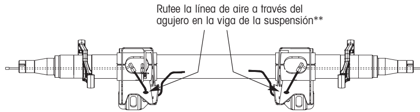
Figura 24. Detalles de instalación sugerida de la línea de control para Modelos Estándar de Perfil Bajo, Buje Ancho (AAL 23K, AAL 25K, AAZL, AAL 30K); Modelos de Servicio Severo de Perfil Bajo, Buje Ancho (AAEDL 30K); y Modelos de Servicio Severo de Montaje por Arriba del Eje, Buje Ancho (AAEDT 30K)
