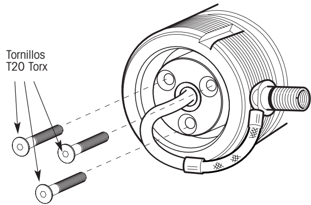
Figura 40. Desensamblaje de la junta rotativa
