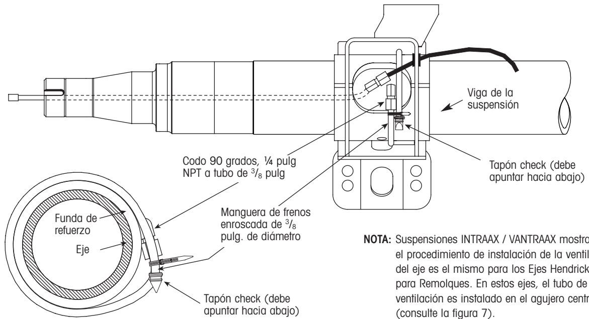
Figura 21. Instalación típica de la manguera de ventilación del eje
