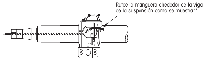
Figura 23. Detalles de instalación sugerida de la línea de control para Modelos Estándar de Montaje por Arriba del Eje, Buje Angosto (HKANT, AANT, AAZNT)
