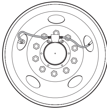
Configuración de llanta dual Orientación "B"
