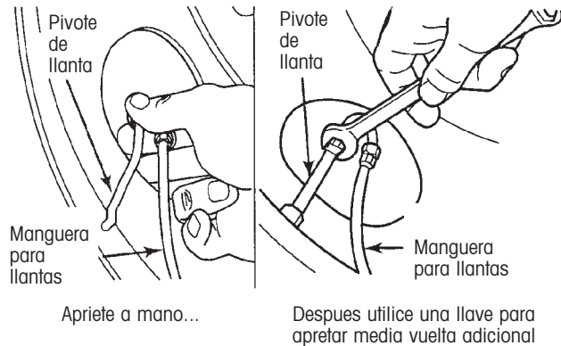
Figura 32. Instale la manguera para llantas en el pivote de la llanta
