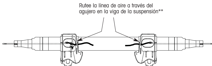
Figura 25a Detalles de instalación sugerida de la línea de control para Modelos Estándar de Perfil Bajo, Buje Angosto (AANL)
