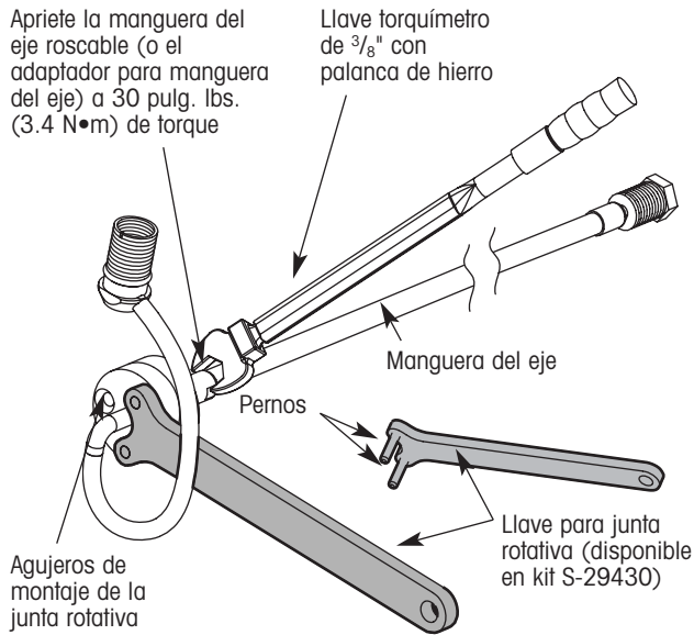
Figura 16. Uso de la llave para junta rotativa
