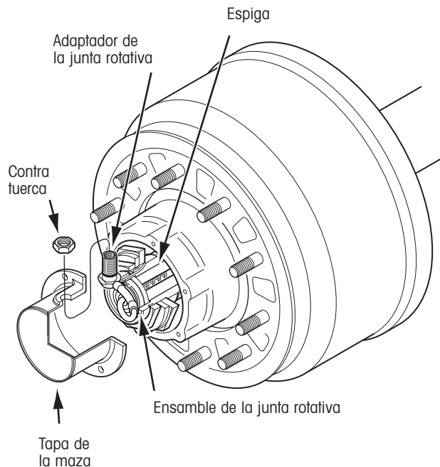
Figura 39. Desensamblaje del adaptador de la junta rotativa
