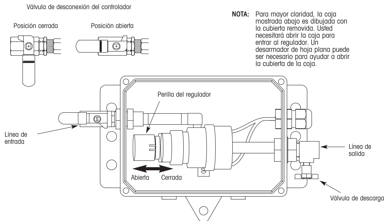
Figura 35. Programación de presión objetivo usando el UCPI
