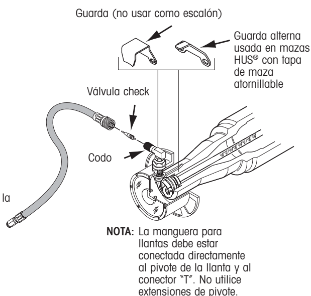
Configuración de llantas sencillas anchas
