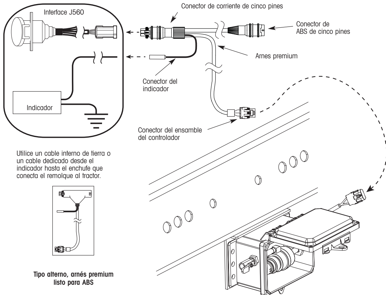
Figura 36. Reemplazo del arnes premium
