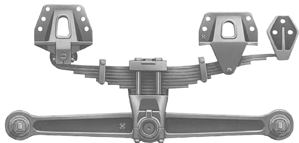
Serie RT con viga de servicio severo
